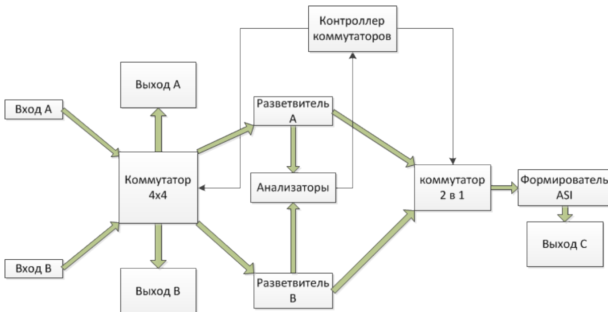
Рис. 1. Прохождение сигнала в РАС-4212
